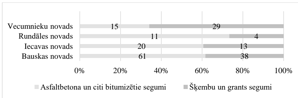
62. attēls. Pašvaldību ielu segums 2020. gadā, km (avots – CSP).
