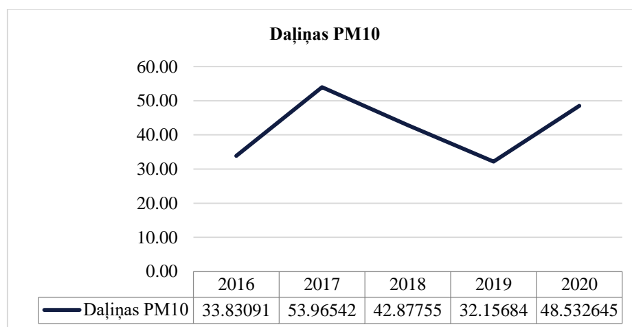
10. attēls. Daļiņu PM10 emisijas t/gadā 2016.-2020, Bauskas novadā (avots – LVĢMC).
