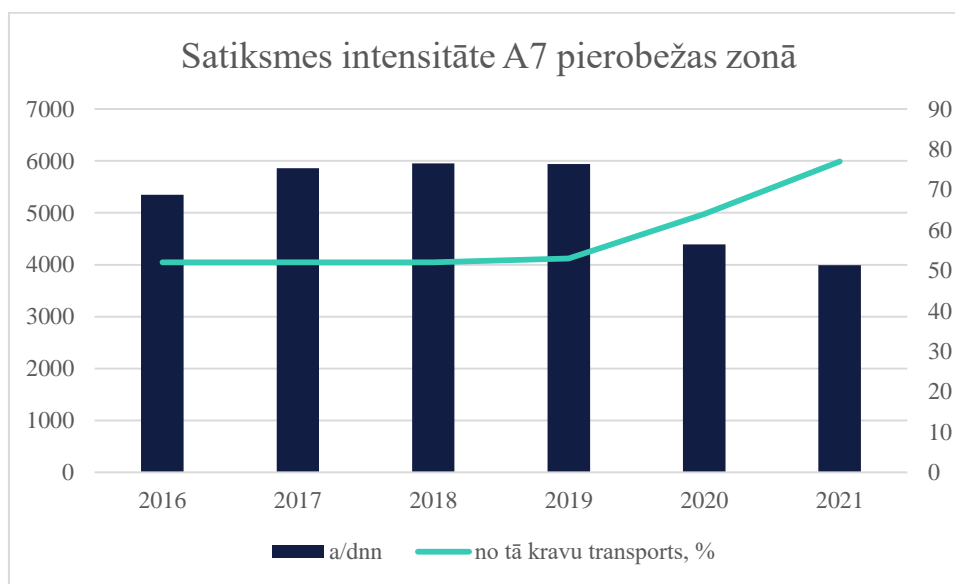
12.attēls. Satiksmes intensitāte A7 pierobežas zonā, LVC 2021..
