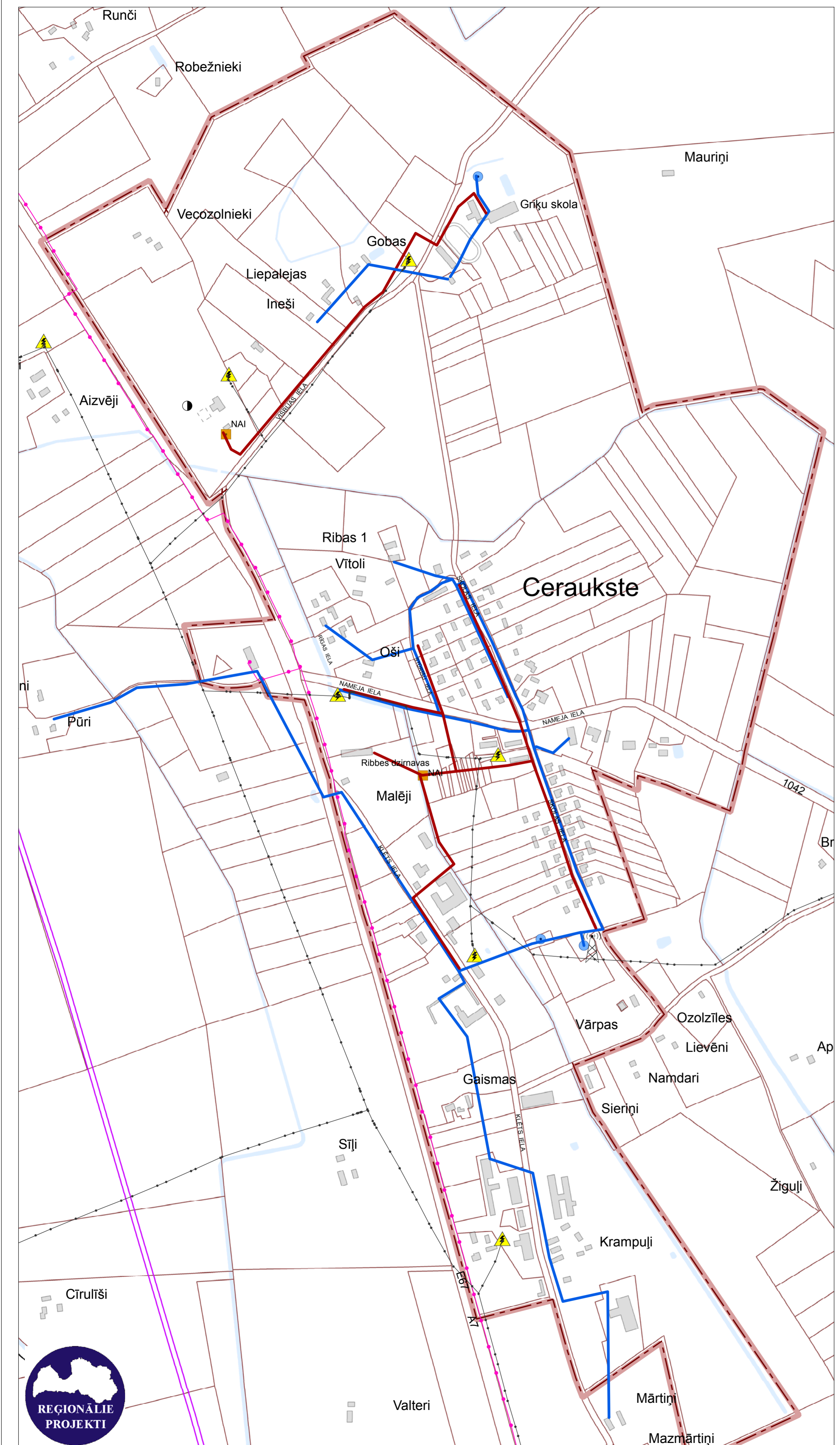
14.kartoshēma. Ceraukstes pagasta ciemu inženiertehniskās apgādes tīkli un objekti. Mērogs 1:5 000
