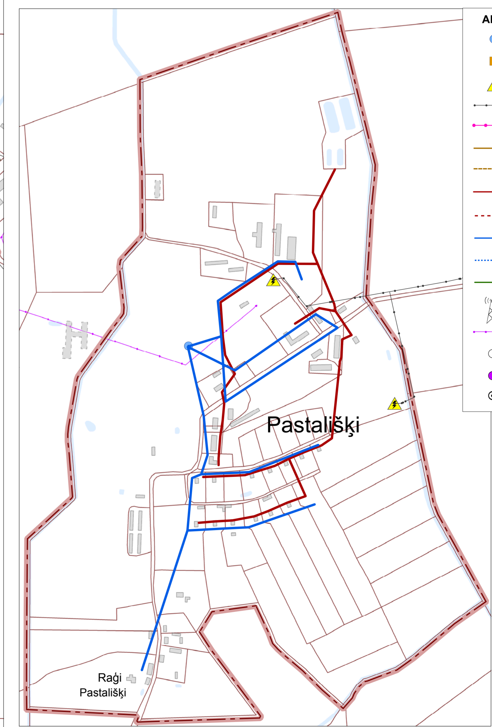
16.kartoshēma. Isītes pagasta ciemu inženiertehniskās apgādes tīkli un objekti. Mērogs 1:5 000
